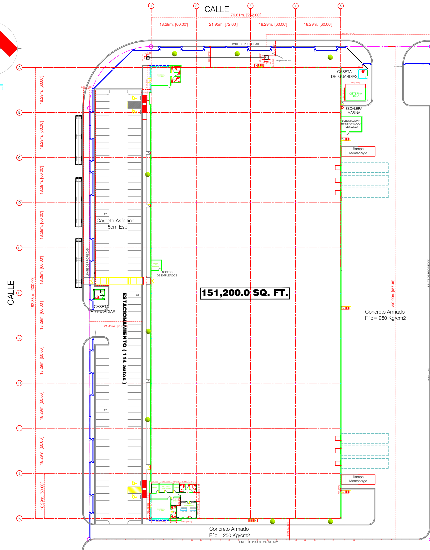
PLANTA ARQUITECTONICA ESC. 1:400
